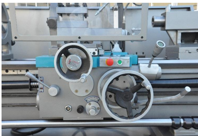
Фартук суппорта (каретка)
