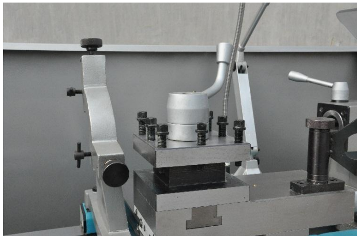
4-позиционный револьверный резцедержатель
