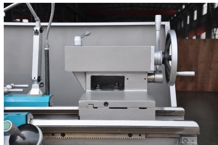
Ручная задняя бабка
